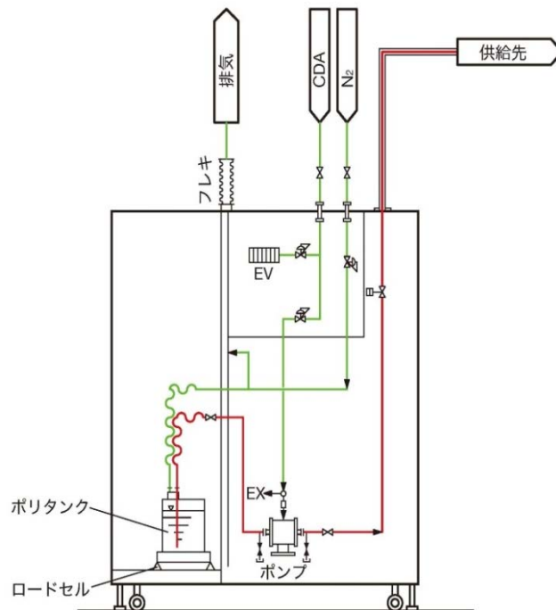
SCSシリーズModel-II フロー図
